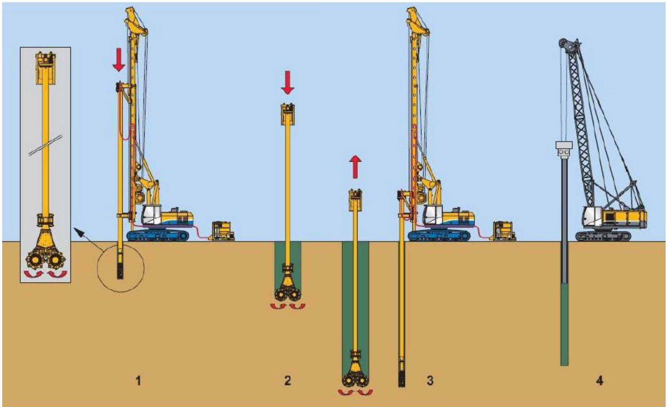
Figura 4-3: Fasi di realizzazione del Cutter Soil Mixing
